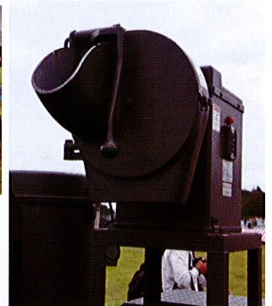
◇写真上は、一度に200人分の主食・副食を調理出来る「野外炊具1号」(22改)、右は切ったり皮を剥いたり珍しい、葉物・球根野菜の便利な調理機具だそうです。
